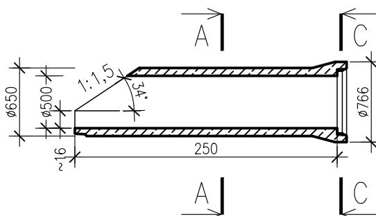
PRZEKRÓJ B-B
